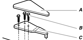
A. Tapa de la bisagra superior B. Tornillos de cabeza hexagonal para bisagra de \frac{5}{16} " C. Bisagra superior
