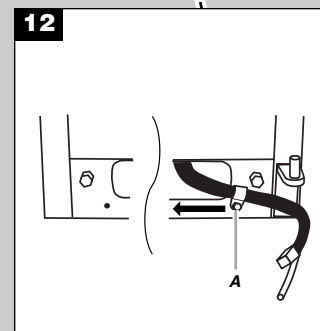
A. Abrazadera de la manguera
