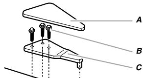
A. Couverture de la charnière supérieure B. Vis de charnière à tête hexagonale de 5/16" C. Charnière supérieure
